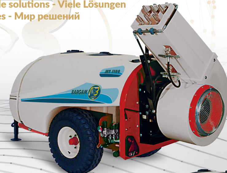
TURBO JET 1100 - 1650 2200 - 3300
